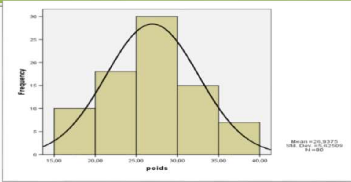
التمثيل البياني للتوزيع التكراري المطلق أو النسبي
