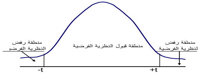
شكل رقم (12): مناطق قبول ورفض النظرية الفرضية
