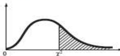
Loi du khi-deux Table de dépassement de l'écart
